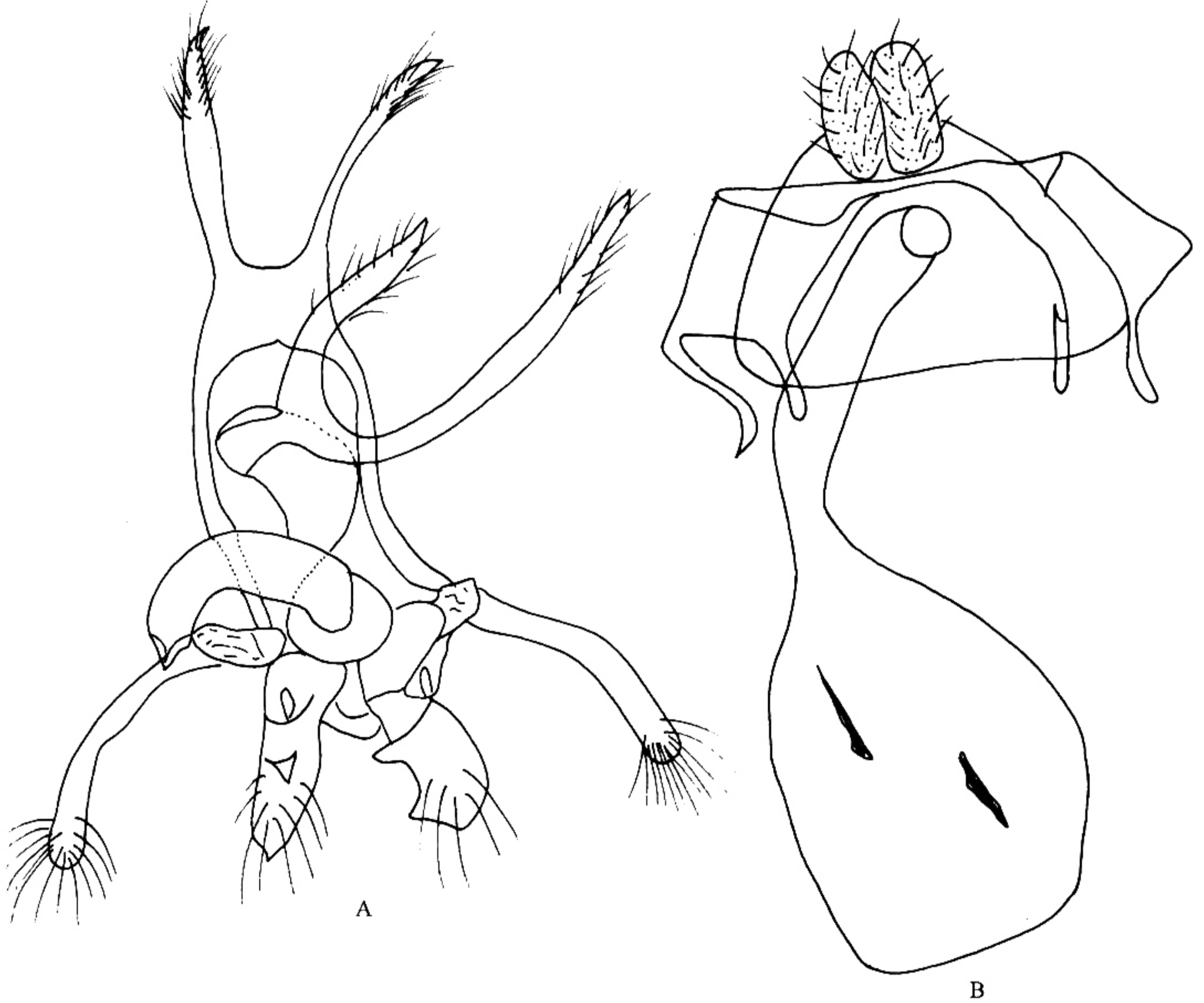
图 156 异纤舟蛾 Periergos ( P. ) dispar (Kiriakoff)
