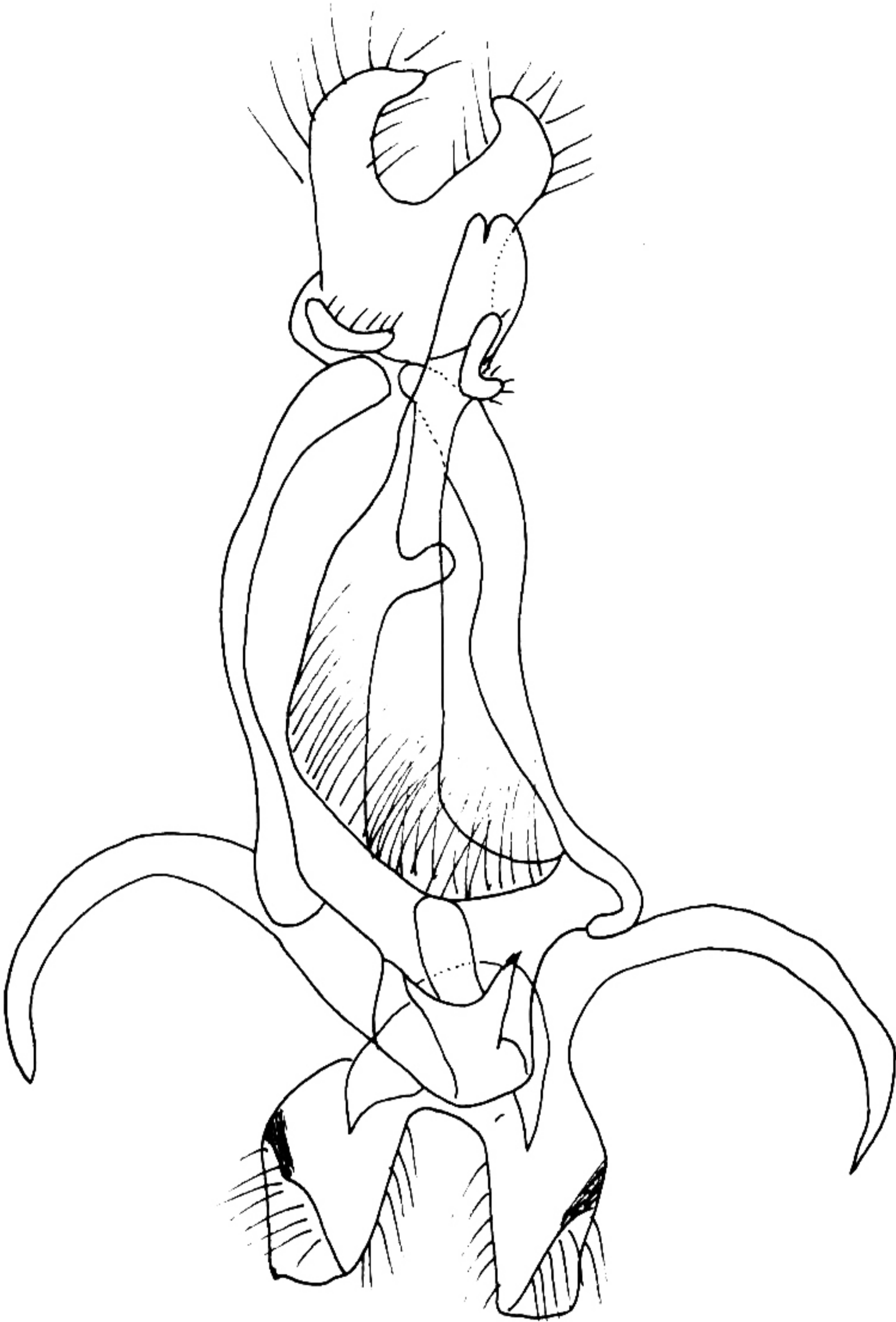
图 155 偶纭舟蛾 Periergos ( P. ) accidentia Schintlmeister et Fang 的雄性外生殖器
